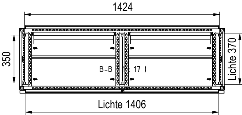
Bodenbefestigung □14mm
