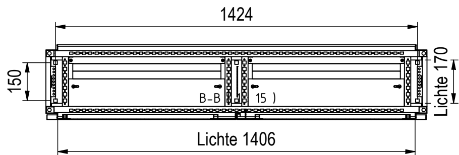
Bodenbefestigung □14mm
