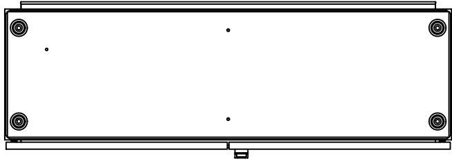
Bodenbefestigung □14mm 1124
