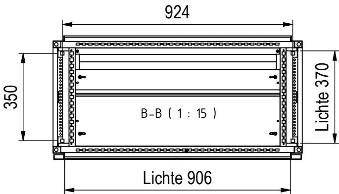
Bodenbefestigung □14mm
