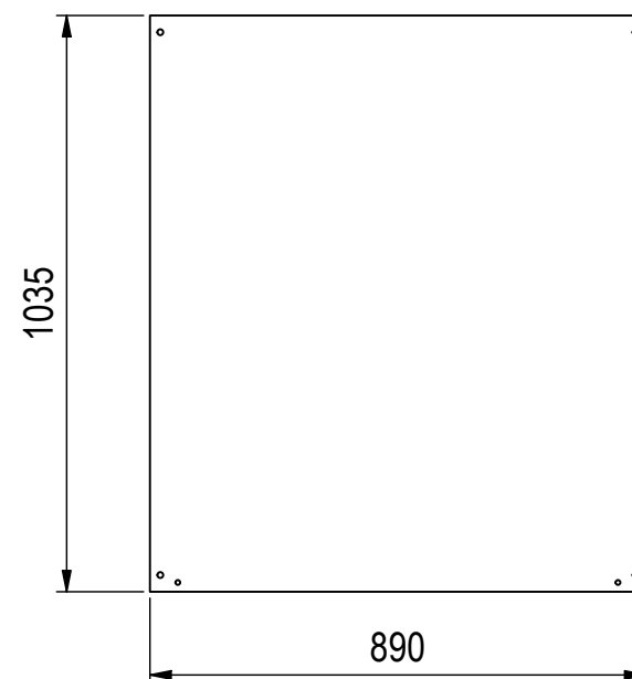
Montageplatte ( 1 : 15 )
