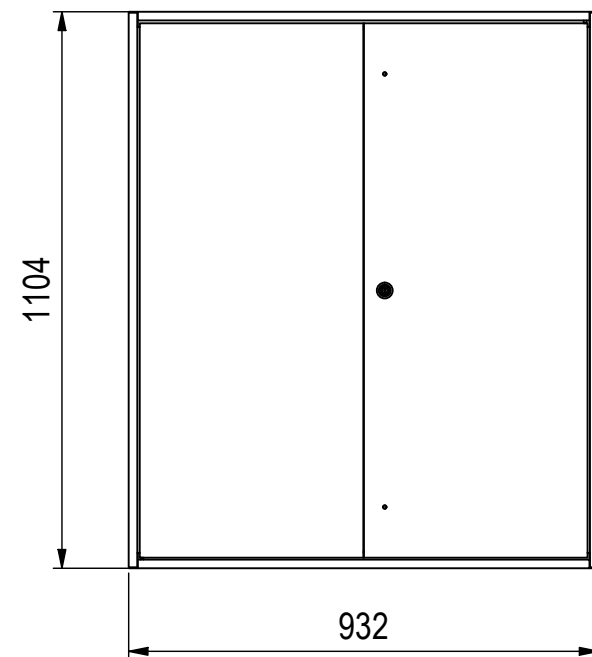
Innenschrank ( 1 : 15 )
