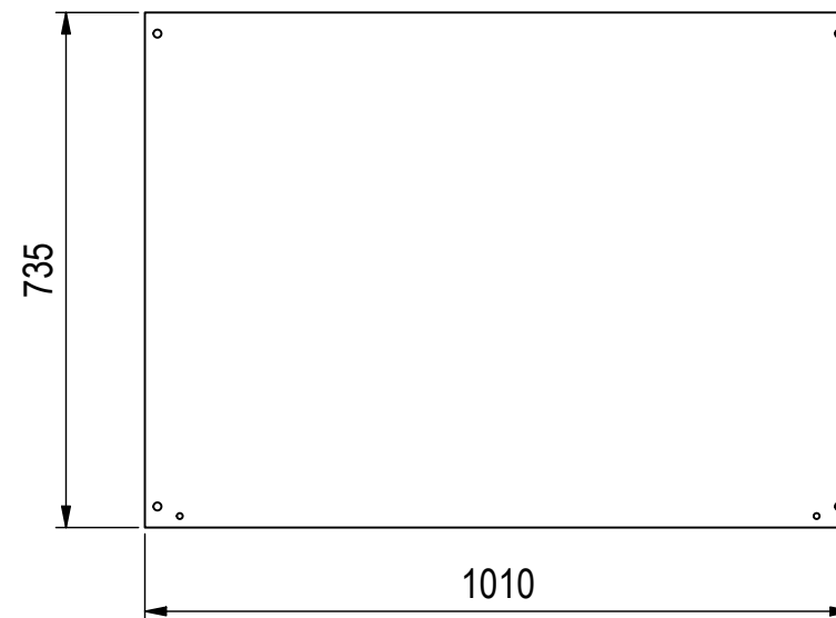
Montageplatte ( 1 : 12 )
