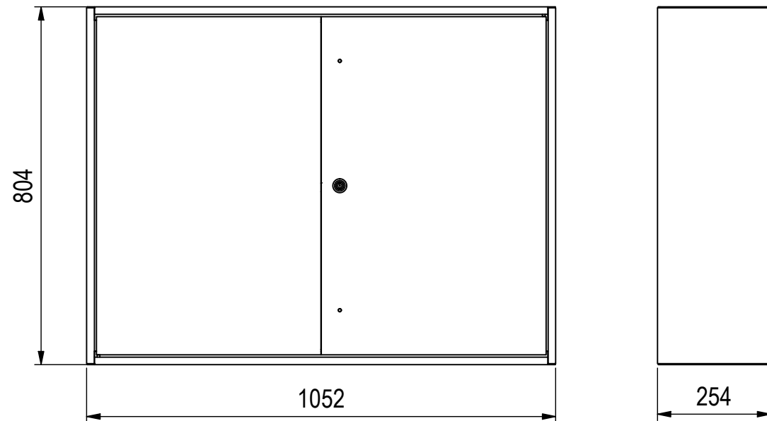
Innenschrank ( 1 : 12 )
