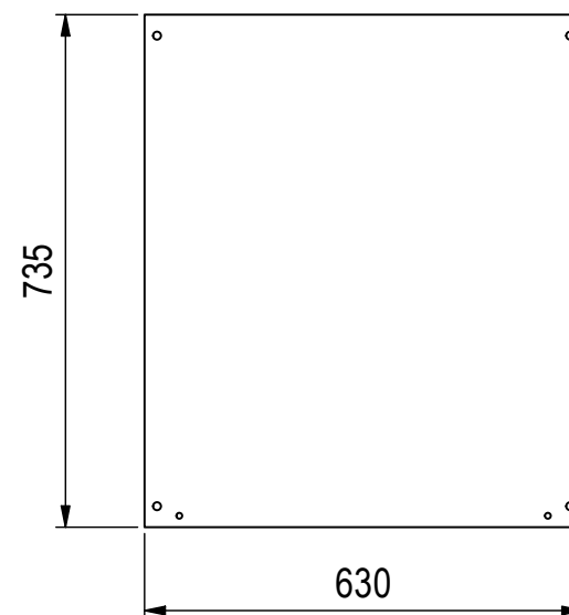
Montageplatte ( 1 : 12 )
