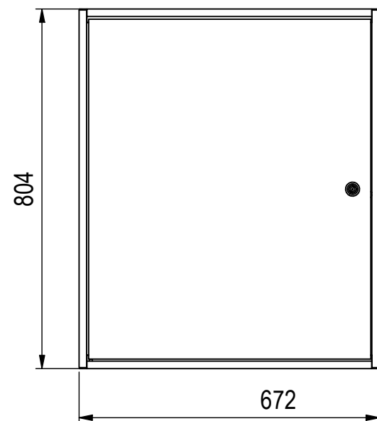
Innenschrank ( 1 : 12 )
