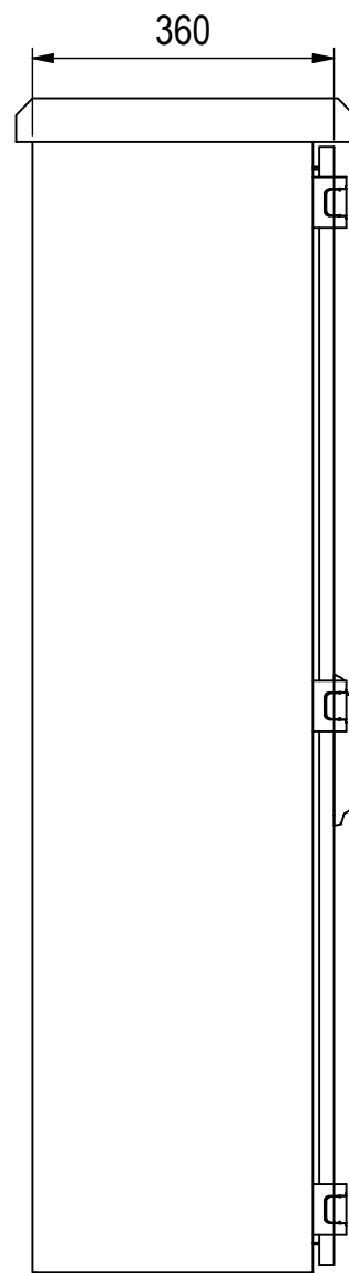
Montageplatte ( 1 : 10 )
