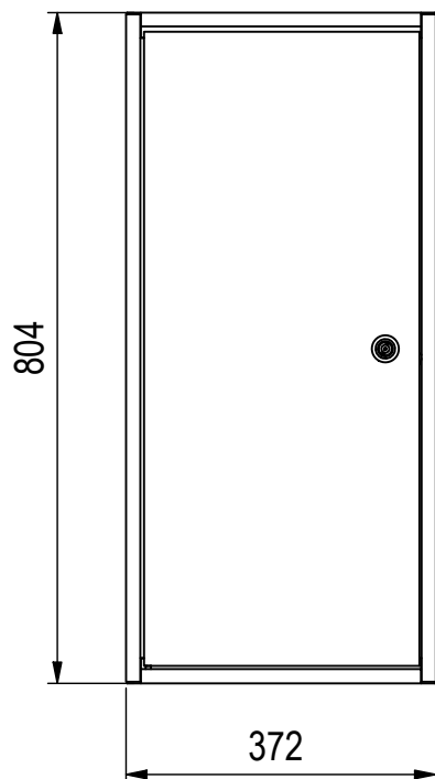
Innenschrank ( 1 : 10 )
