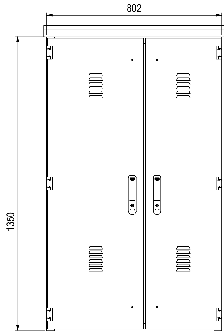
Innenschrank ( 1 : 10 )
