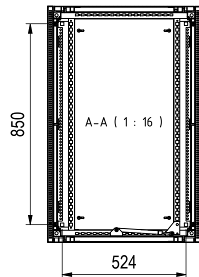
Bodenbefestigung □14mm
