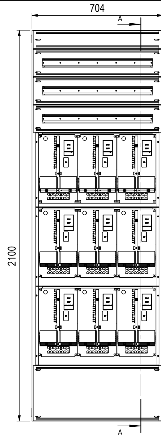
Hutschiene Vorzählerfach 629
