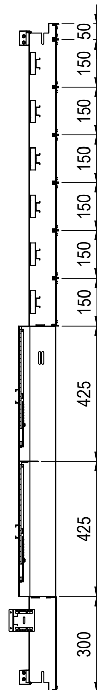
A-A ( 1 : 12 )
