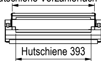
Hutschiene Vorzählerfach 429
