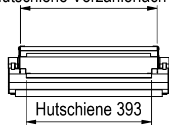
Hutschiene Vorzählerfach 429
