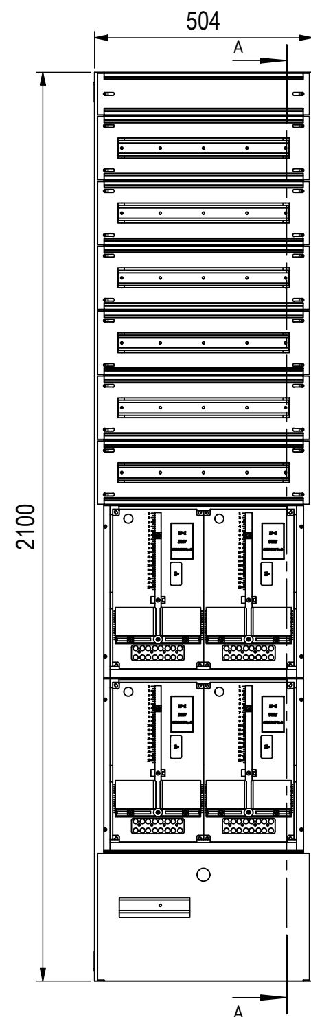
Hutschiene Vorzählerfach 429
