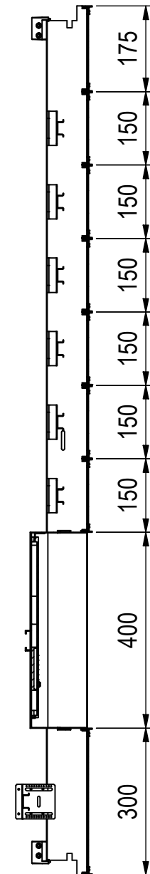
A-A ( 1 : 11 )
