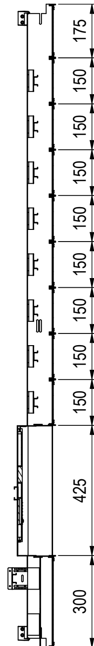
A-A ( 1 : 12 )
