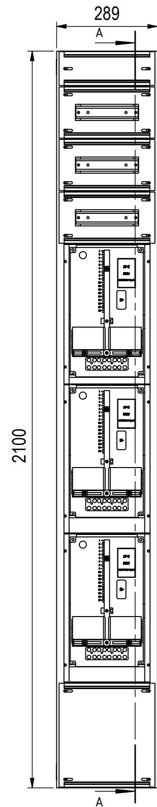
Hutschiene Vorzählerfach 214
