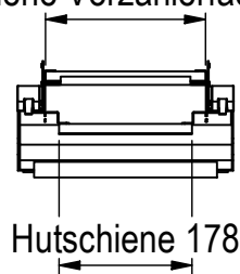
Hutschiene Vorzählerfach 214
