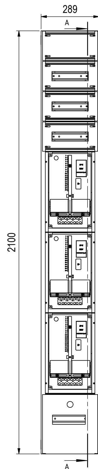
Hutschiene Vorzählerfach 214
