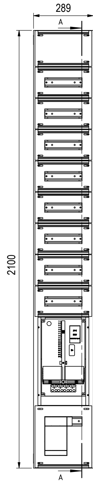
Hutschiene Vorzählerfach 214
