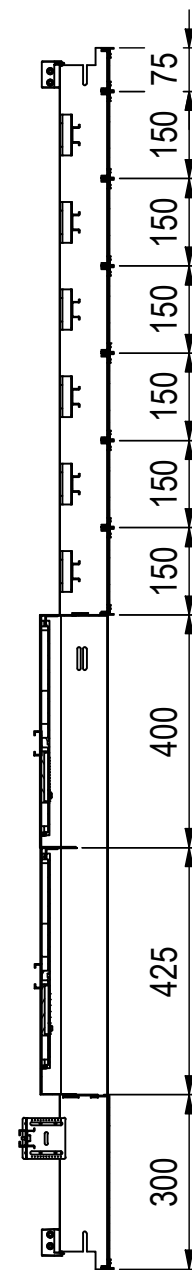
A-A ( 1 : 13 )
