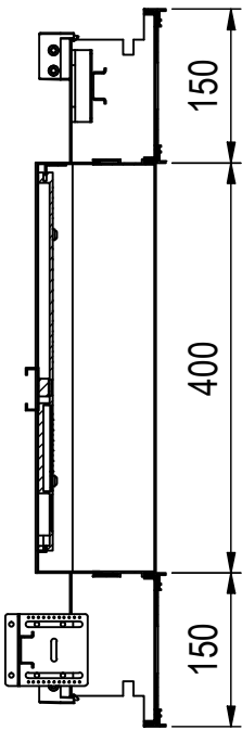
A-A ( 1 : 8 )
