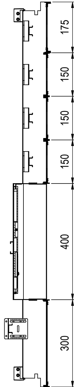
A-A ( 1 : 8 )
