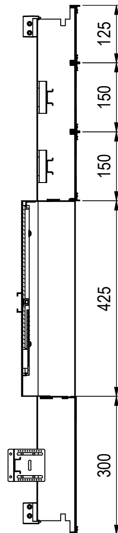
A-A ( 1 : 8 )
