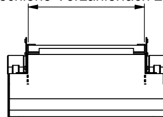
Hutschiene Vorzählerfach 214
