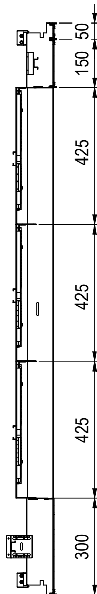
A-A ( 1 : 12 )
