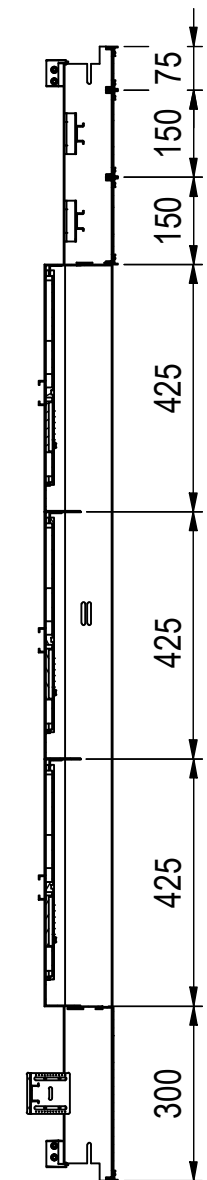
A-A ( 1 : 13 )
