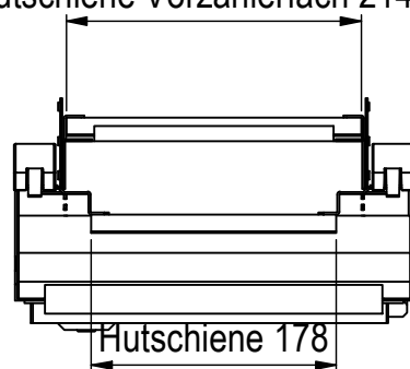
Hutschiene Vorzählerfach 214
