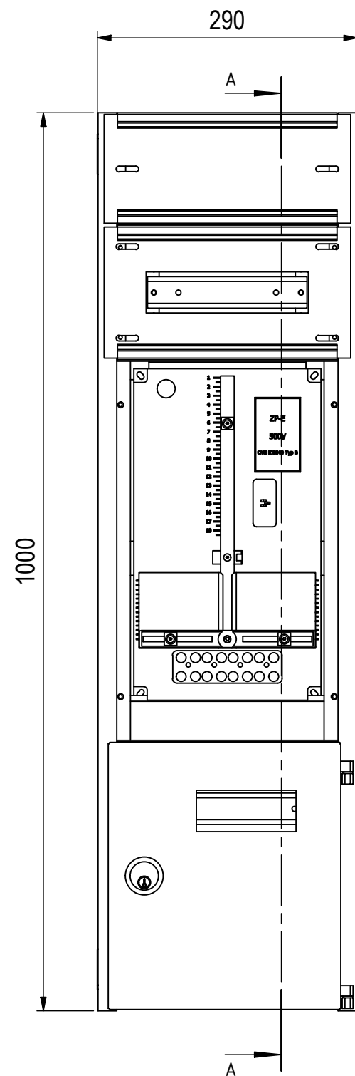
Hutschiene Vorzählerfach 214
