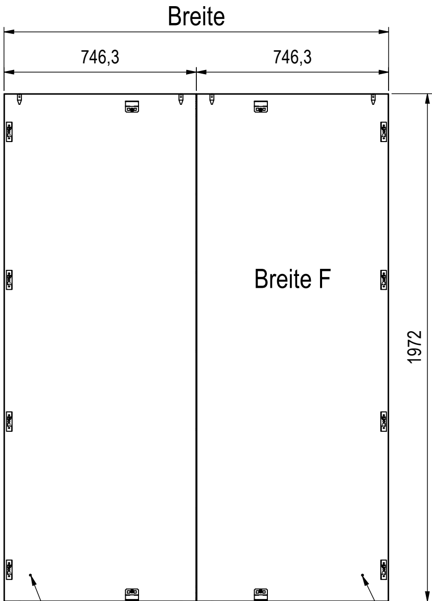
Erdungsbolzen M6x16
