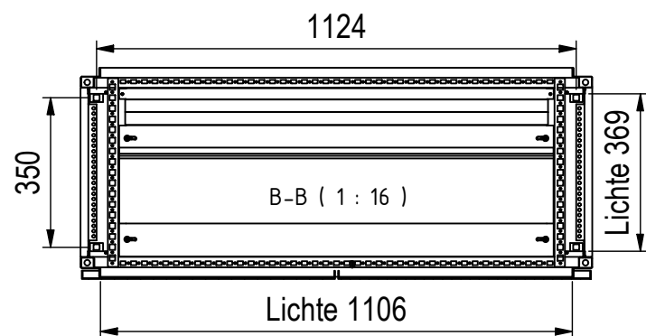
Bodenbefestigung □14mm
