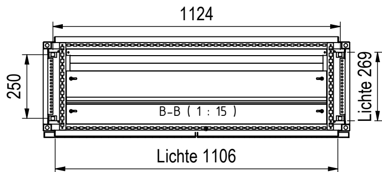
Bodenbefestigung □14mm
