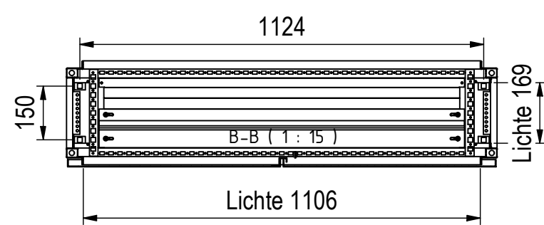
Bodenbefestigung □14mm
