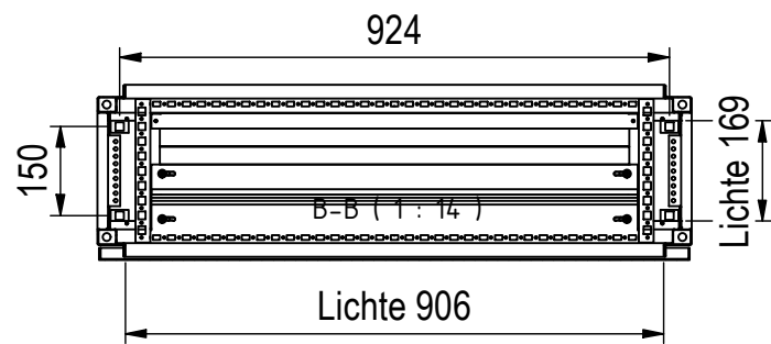
Bodenbefestigung □14mm
