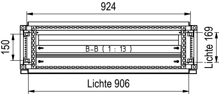
Bodenbefestigung □14mm
