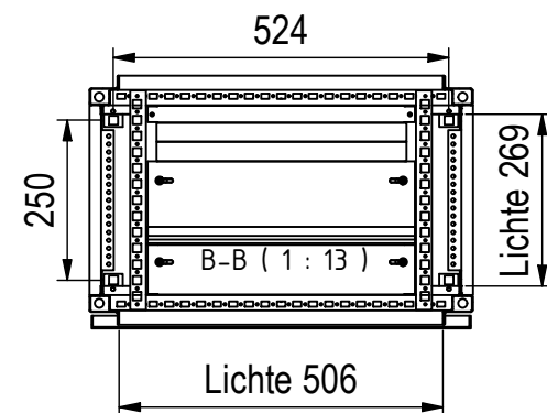
Bodenbefestigung □14mm
