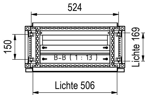
Bodenbefestigung □14mm
