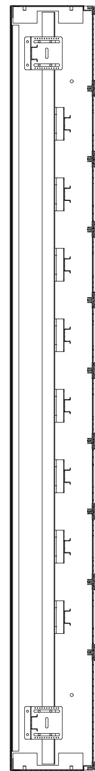
D-D ( 1 : 8 )
