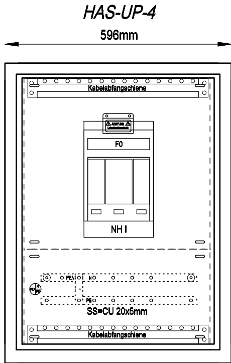
Frontansicht ohne Tür
