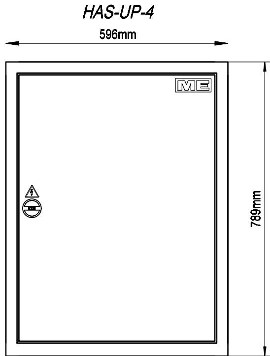
Frontansicht mit Tür
