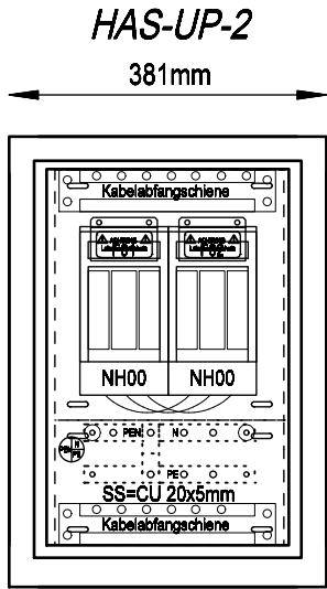
Frontansicht ohne Tür
