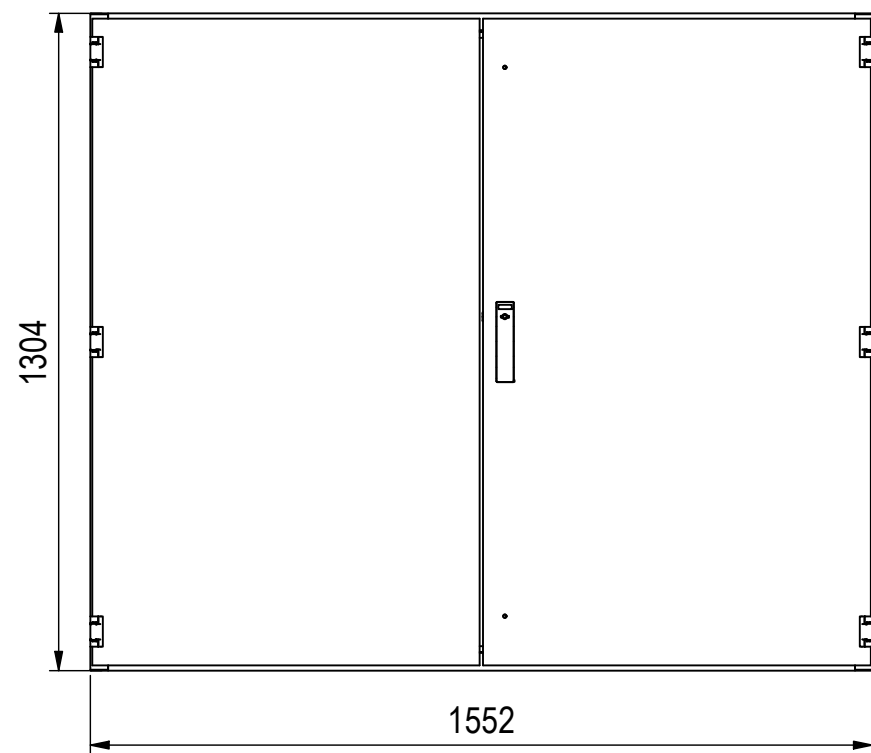
Innenschrank ( 1 : 15 )
