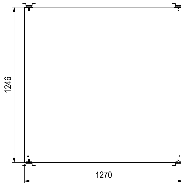
Montageplatte ( 1 : 15 )
