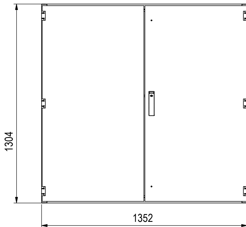
Innenschrank ( 1 : 15 )
