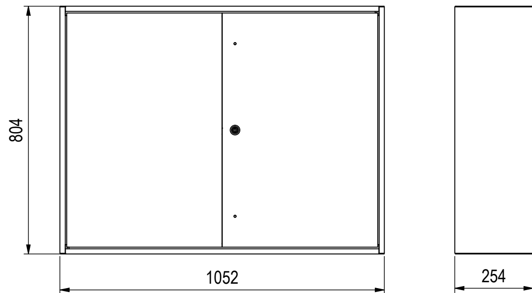
Innenschrank ( 1 : 12 )
