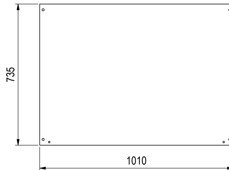
Montageplatte ( 1 : 12 )
