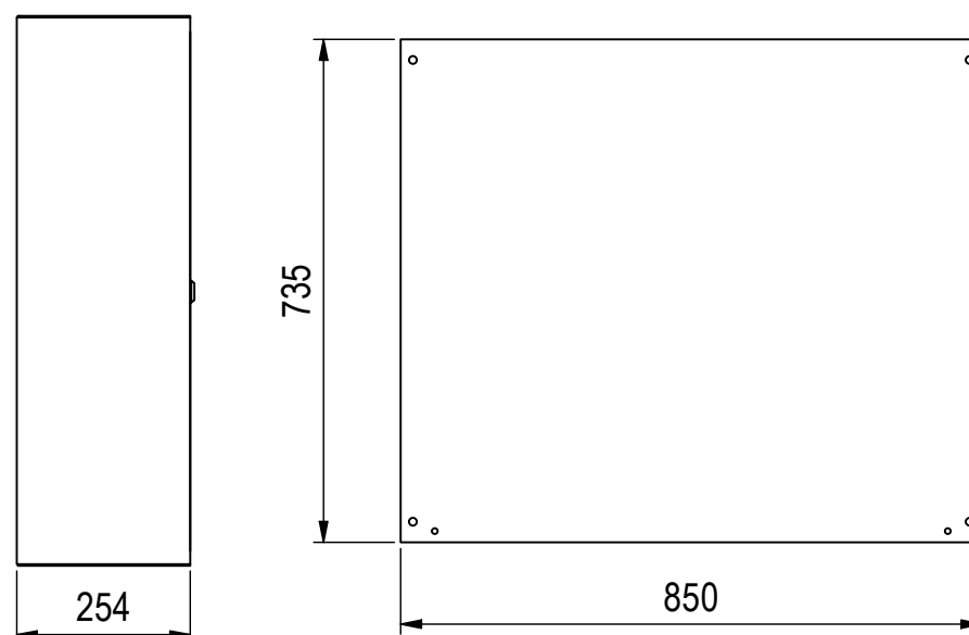
Montageplatte ( 1 : 12 )
