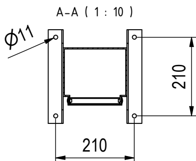
Montageplatte
