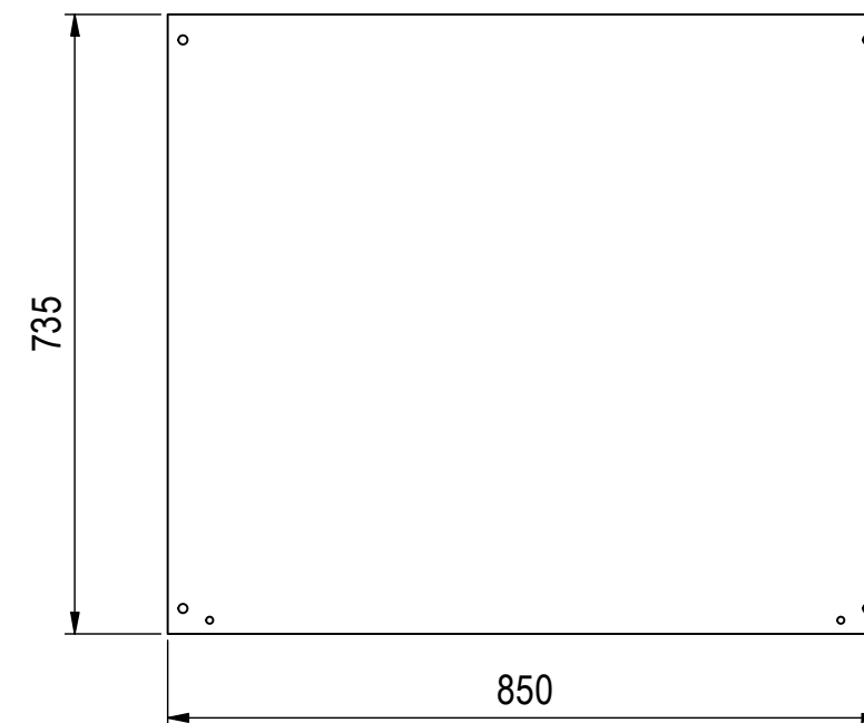
Montageplatte ( 1 : 10 )
