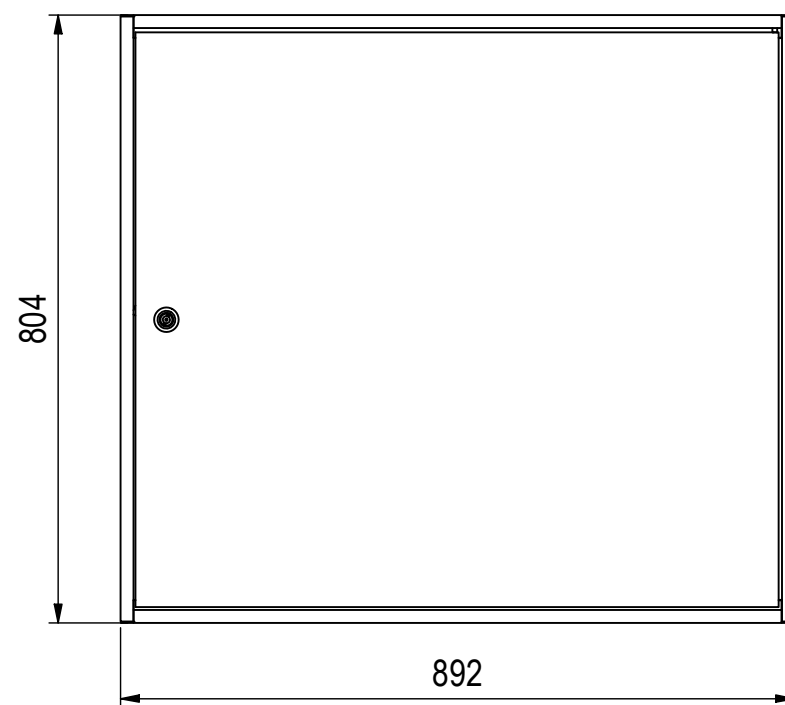
Innenschrank ( 1 : 10 )
