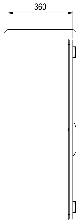
Innenschrank ( 1 : 10 )
