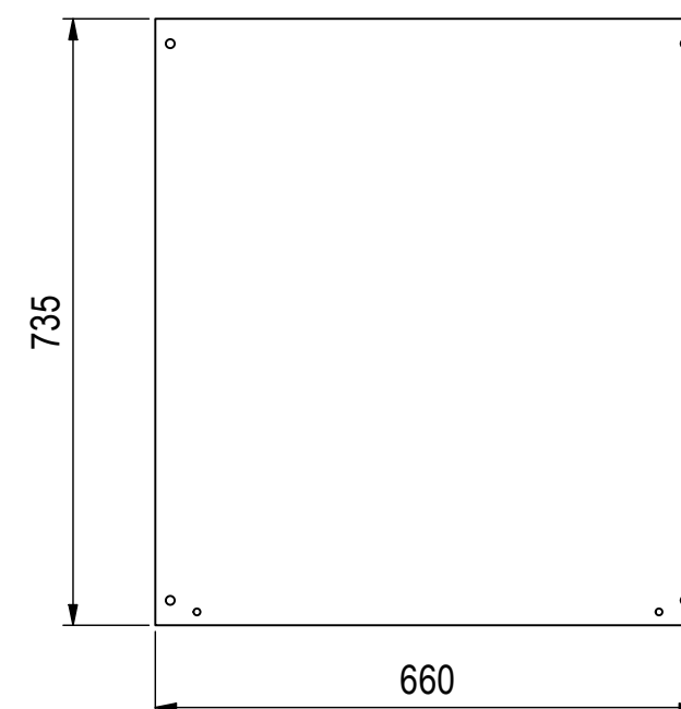
Montageplatte ( 1 : 10 )
