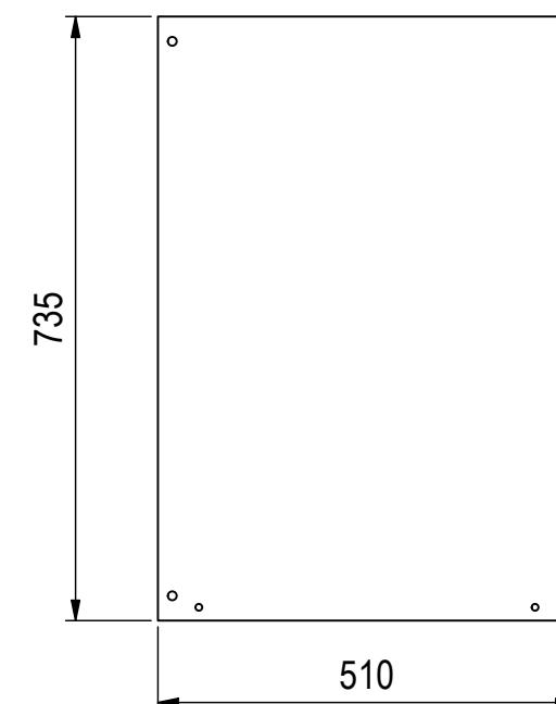
Montageplatte ( 1 : 10 )
