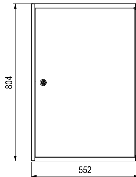
Innenschrank ( 1 : 10 )
