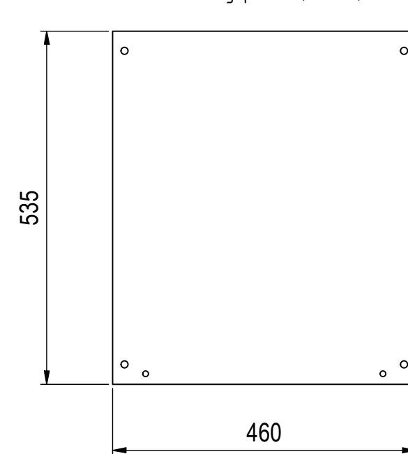
Montageplatte ( 1 : 8 )
