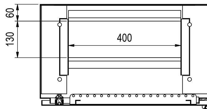
B-B ( 1 : 8 )
