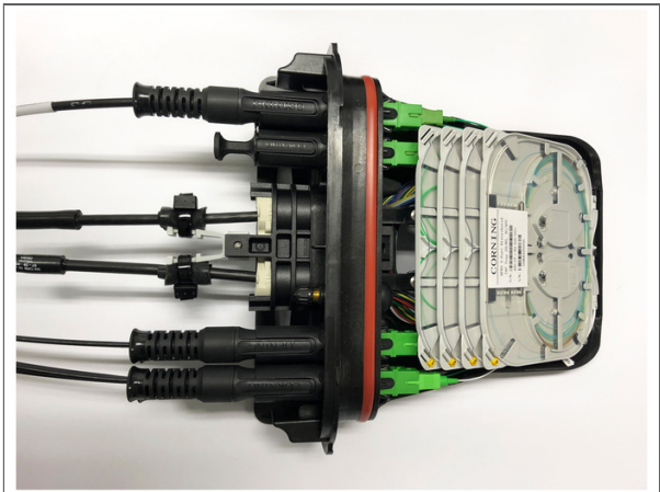
BPEO Glasfasermuffe, Größe 0, mit Evolv Pushlok Technologie, 8 Kabeleinführungen mit 2 Spleißkassetten, 8 SC APC Adapter
